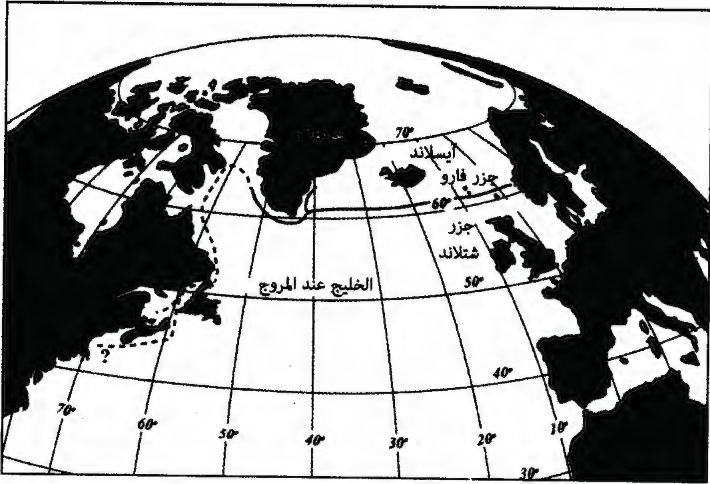
الشكل (1): طرق النورديين من النرويج إلى مستوطنات في غرينلاند (خط متصل)، وطريق ليف إيريكسون المحتمل إلى أمريكا الشمالية (خط منقط) نحو القرن الحادي عشر الميلادي.
